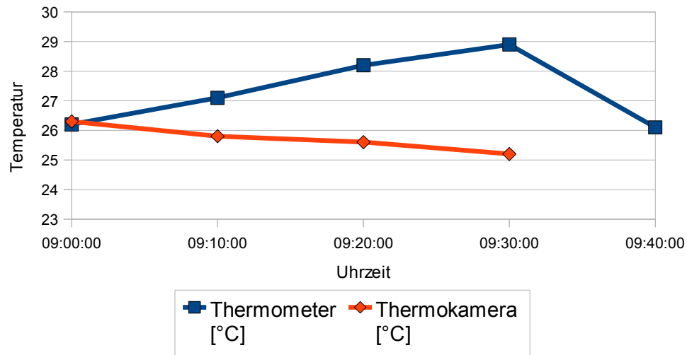
Temperaturverlauf bei unterbrochenem Luftstrom
